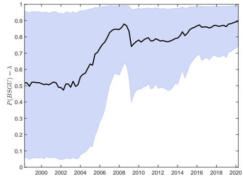
(d) Zero correlations
